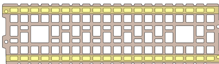
4. Appliquer les cordons de colle sur des blocs propres et dépoussiérés. (2 cordons horizontaux par briques en suivant les rangées d'alvéoles jouxtant les parois extérieurs)
